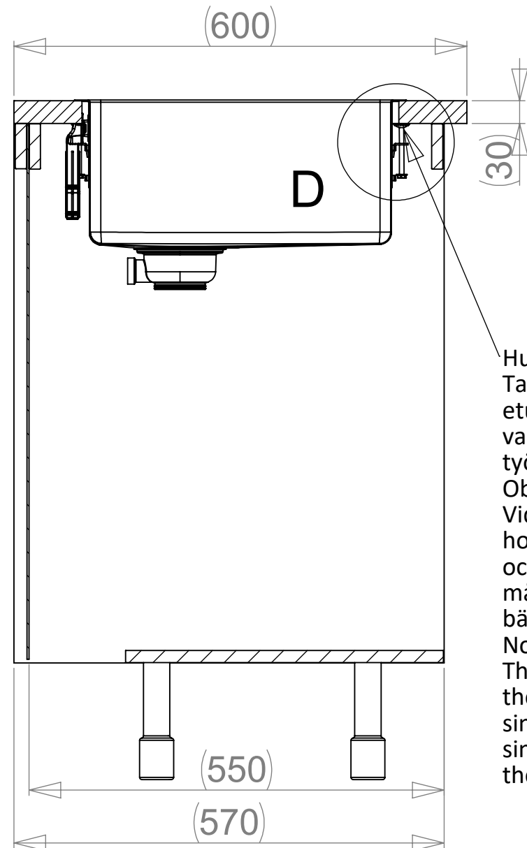
C-C (1 : 7)
